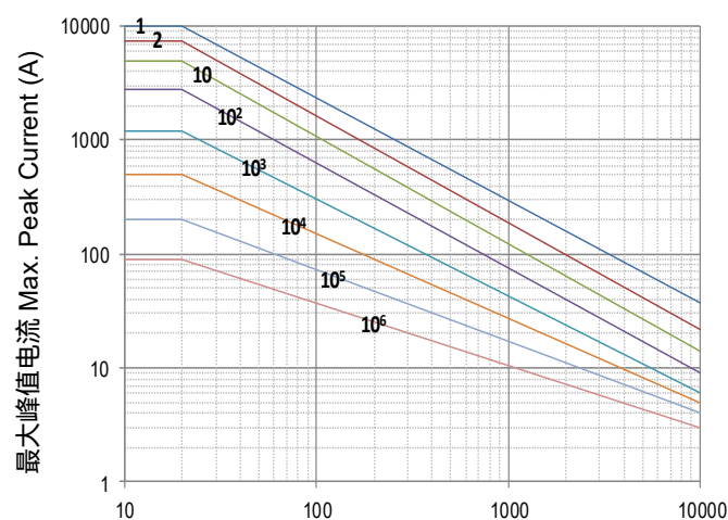
脉冲持续时间 Impulse Duration ( \mu s) SFV15S820K to SFV15S821K
