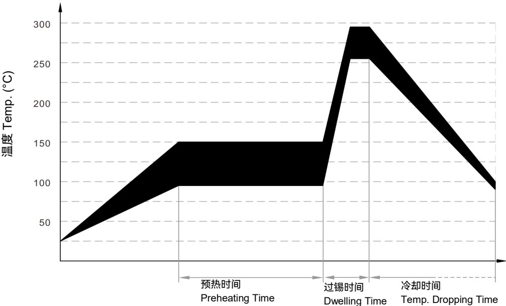
波峰焊曲线 Wave Soldering Curve
